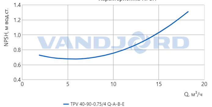
Характеристика NPSH
