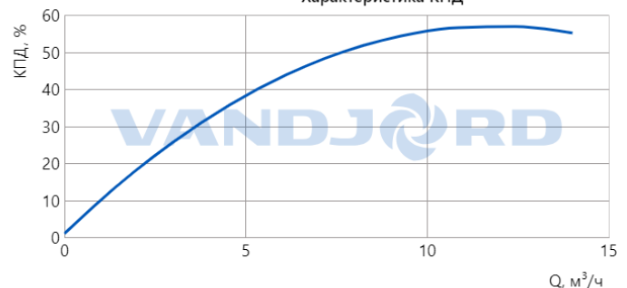
Характеристика КПД
