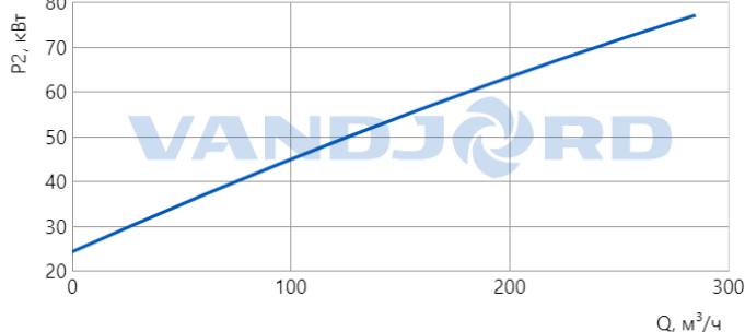
Характеристика мощности
