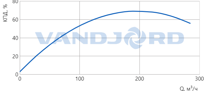
Характеристика КПД
