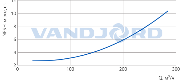
Характеристика NPSH
