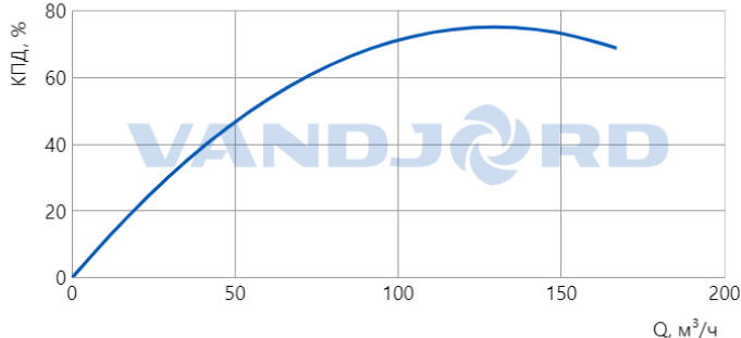
Характеристика КПД
