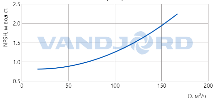
Характеристика NPSH
