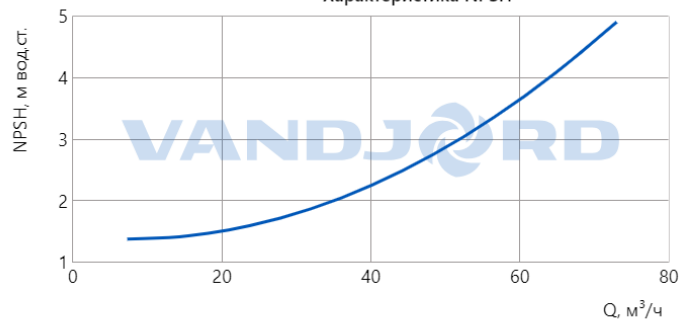
Характеристика NPSH
