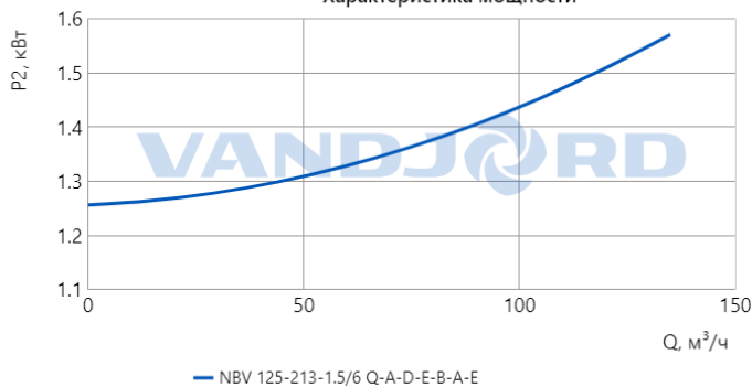
Характеристика мощности
