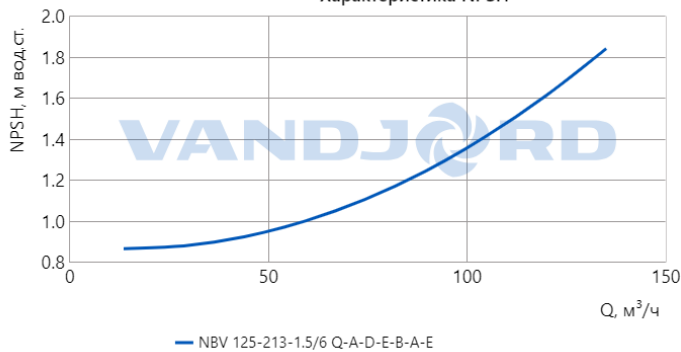
Характеристика NPSH
