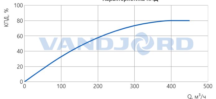
Характеристика КПД
