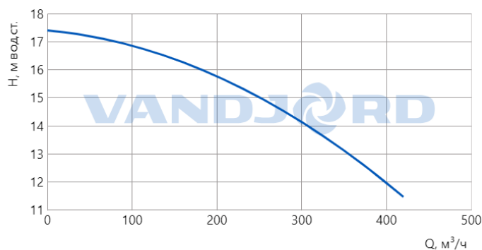
73219026 - NBV 200-337-18.5/6 Q-A-D-E-B-A-E Гидравлическая характеристика
