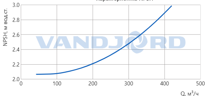
Характеристика NPSH
