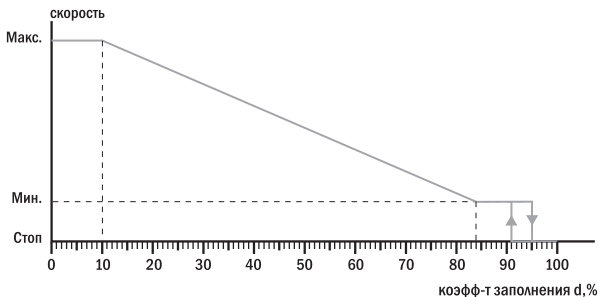
Рис. 12 Зависимость скорости от коэффициента заполнения
