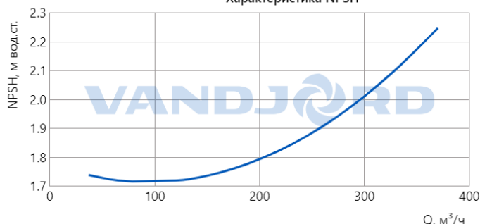
Характеристика NPSH
