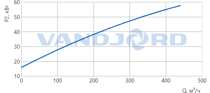
Характеристика мощности
