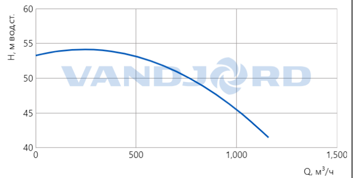
Гидравлическая характеристика
