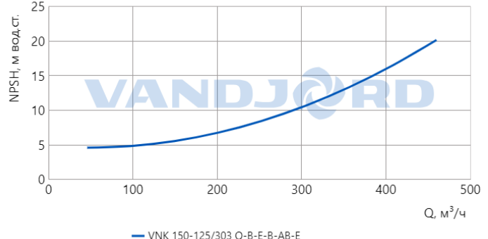
Характеристика NPSH
