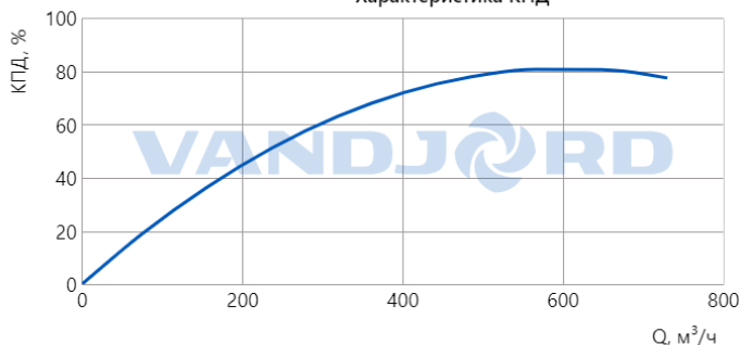
Характеристика КПД
